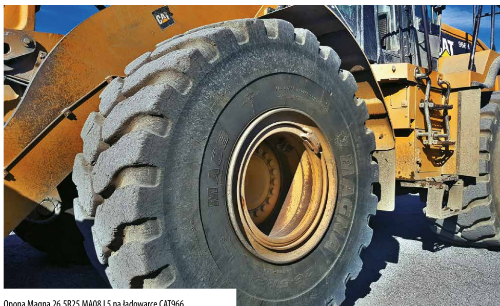
Opona Magna 26,5R25 MA08 L5 na ładowarce CAT966
